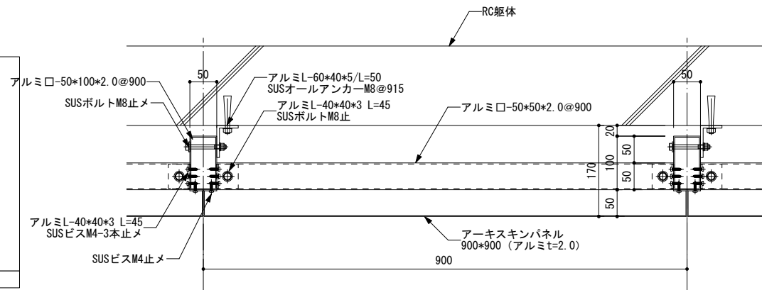
平断面詳細図 (RC) S=1/10
